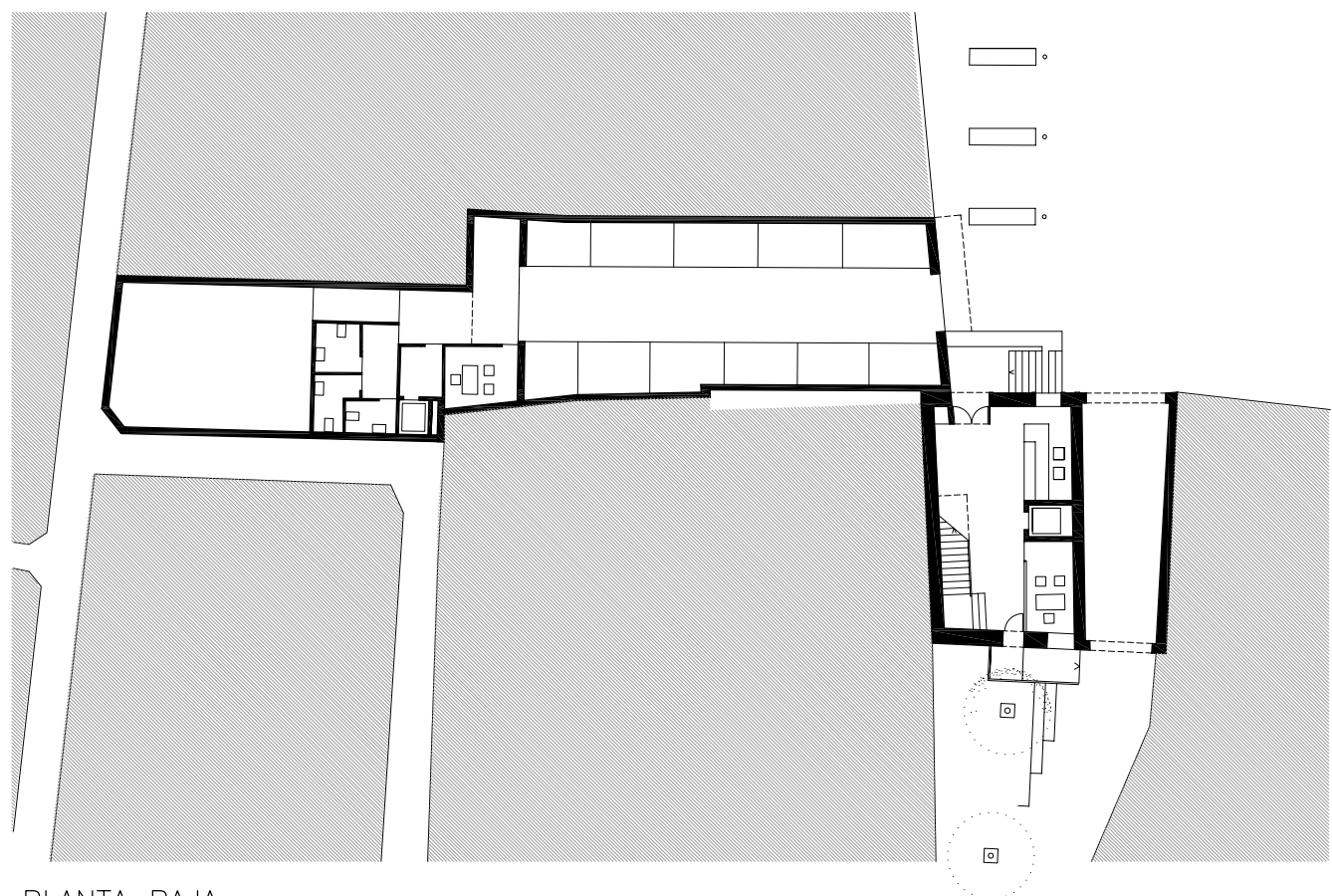
PLANTA BAJA
