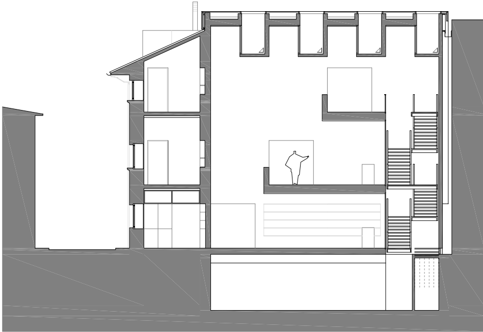
1. SECCIÓN TRANSVERSAL
