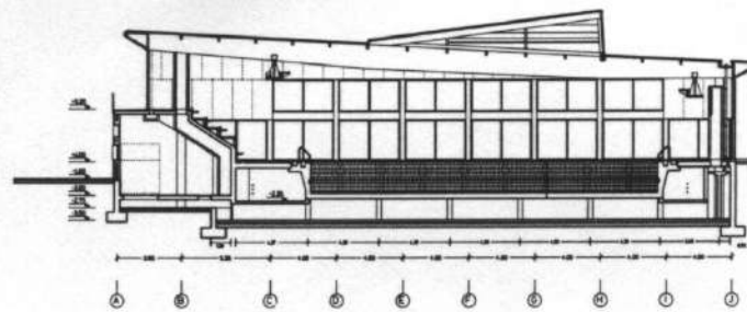
SECCION TRANSVERSAL B - B
