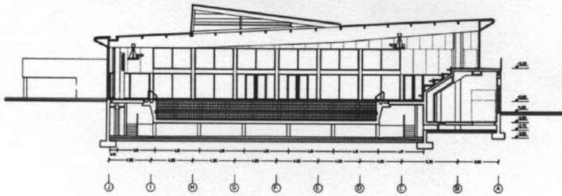
SECCION TRANSVERSAL A - A
