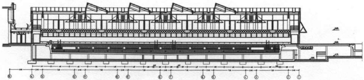
SECCION LONGITUDINAL C - C
