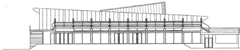
FACHADA-SECCION NORTE ( ANTIGUA PISCINA CUBIERTA)
