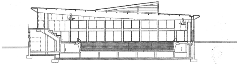
SECCION TRANSVERSAL B - B
