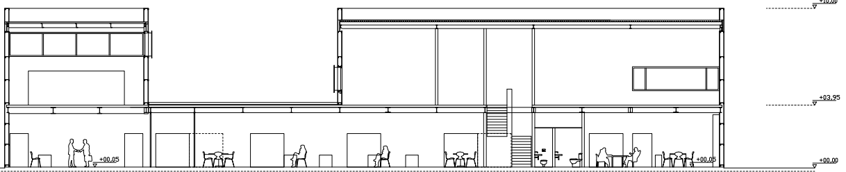
SECCIÓN F-F'
