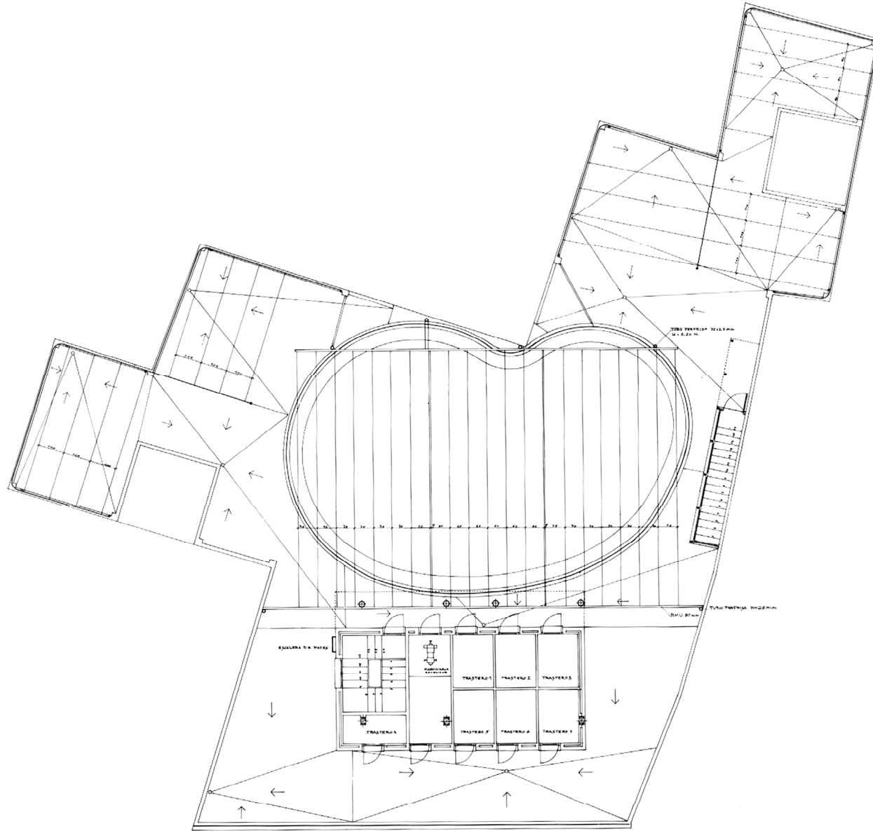
Planta cubierta Bloque de Viviendas en calle Doña María Coronel, Sevilla Cruz y Ortiz arquitectos
