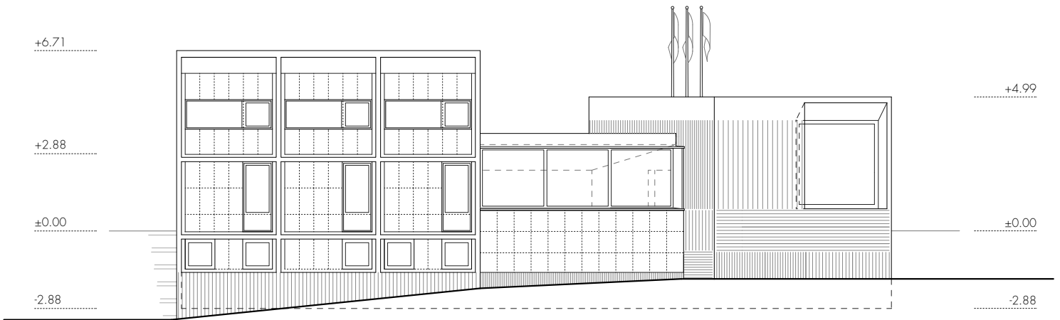
ALZADO SUR
