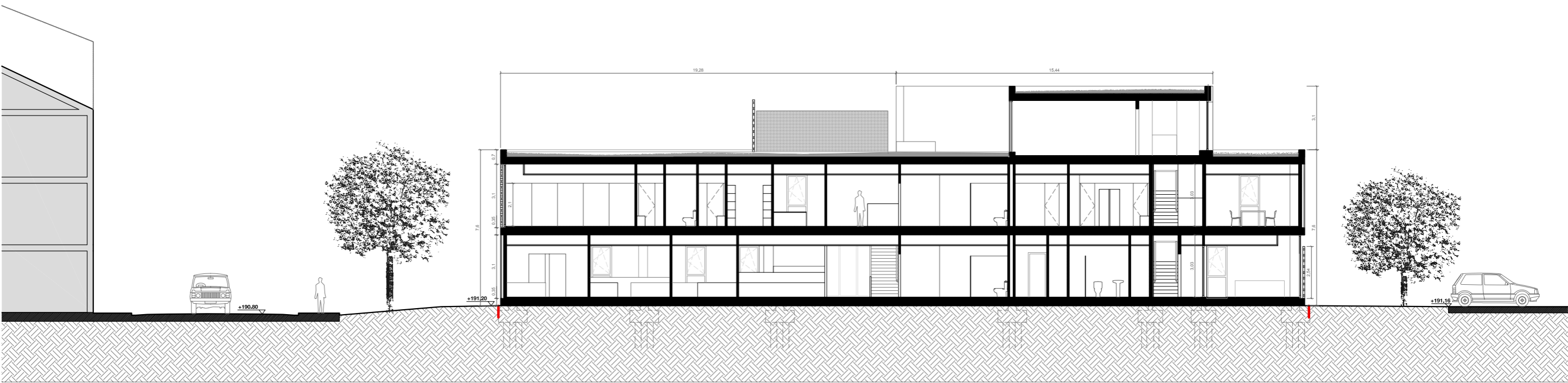
SECCIÓ S2
