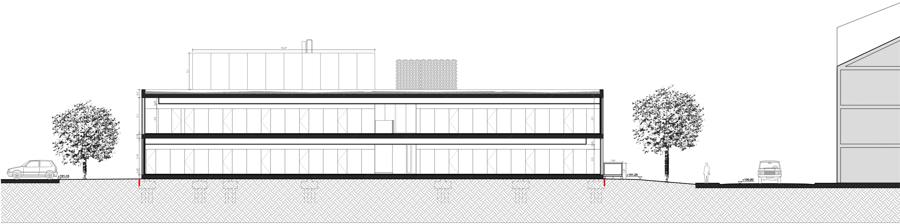
SECCIÓ S1
