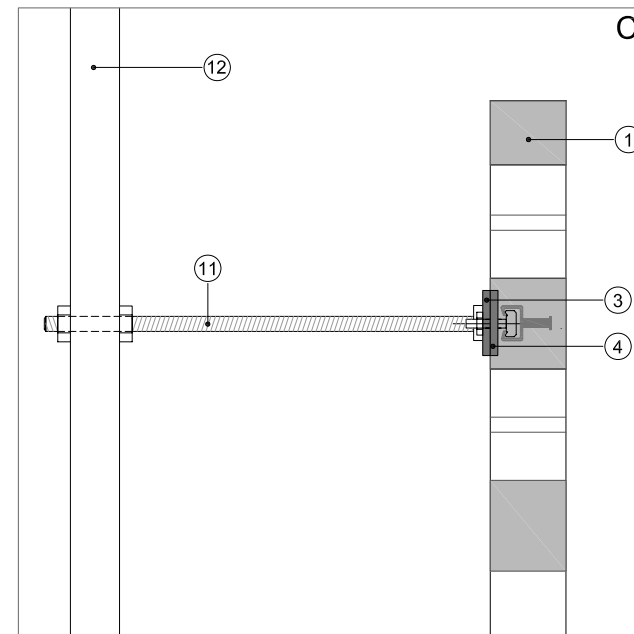
GEOMETRIA GELOSIA PREFABRICADA
