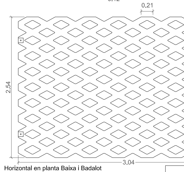
GEOMETRIA GELOSIA PREFABRICADA
