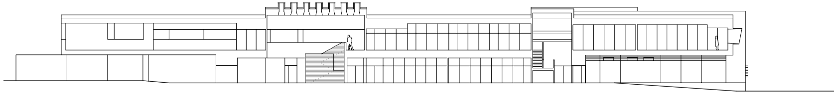
SECCION LONGITUDINAL
