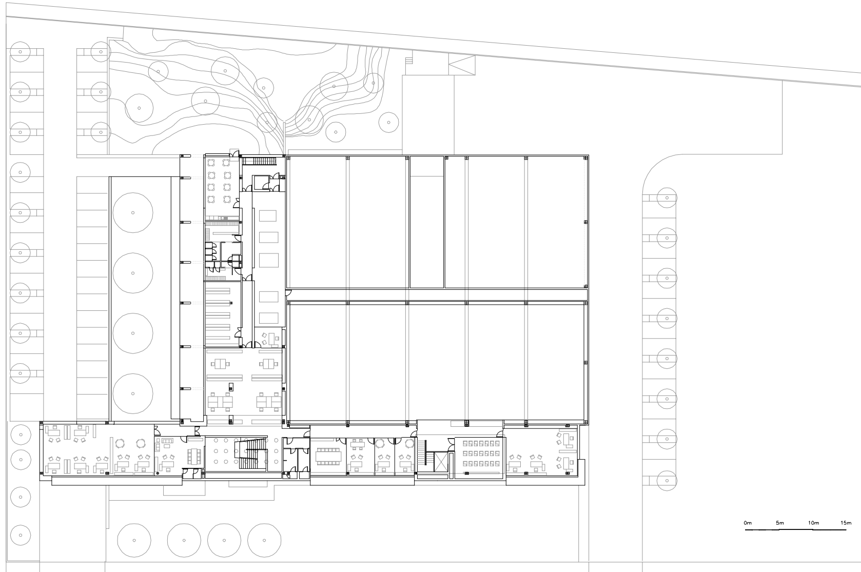
PLANTA PRIMERA
