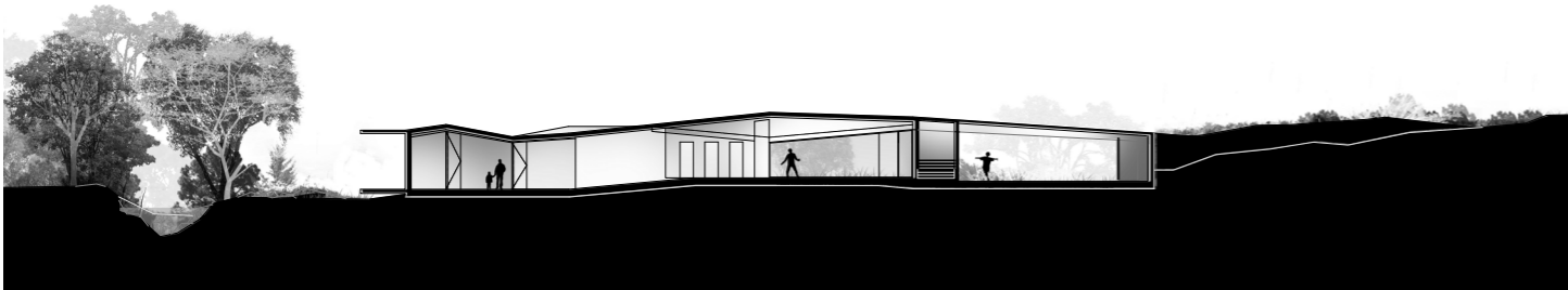
sección 1
