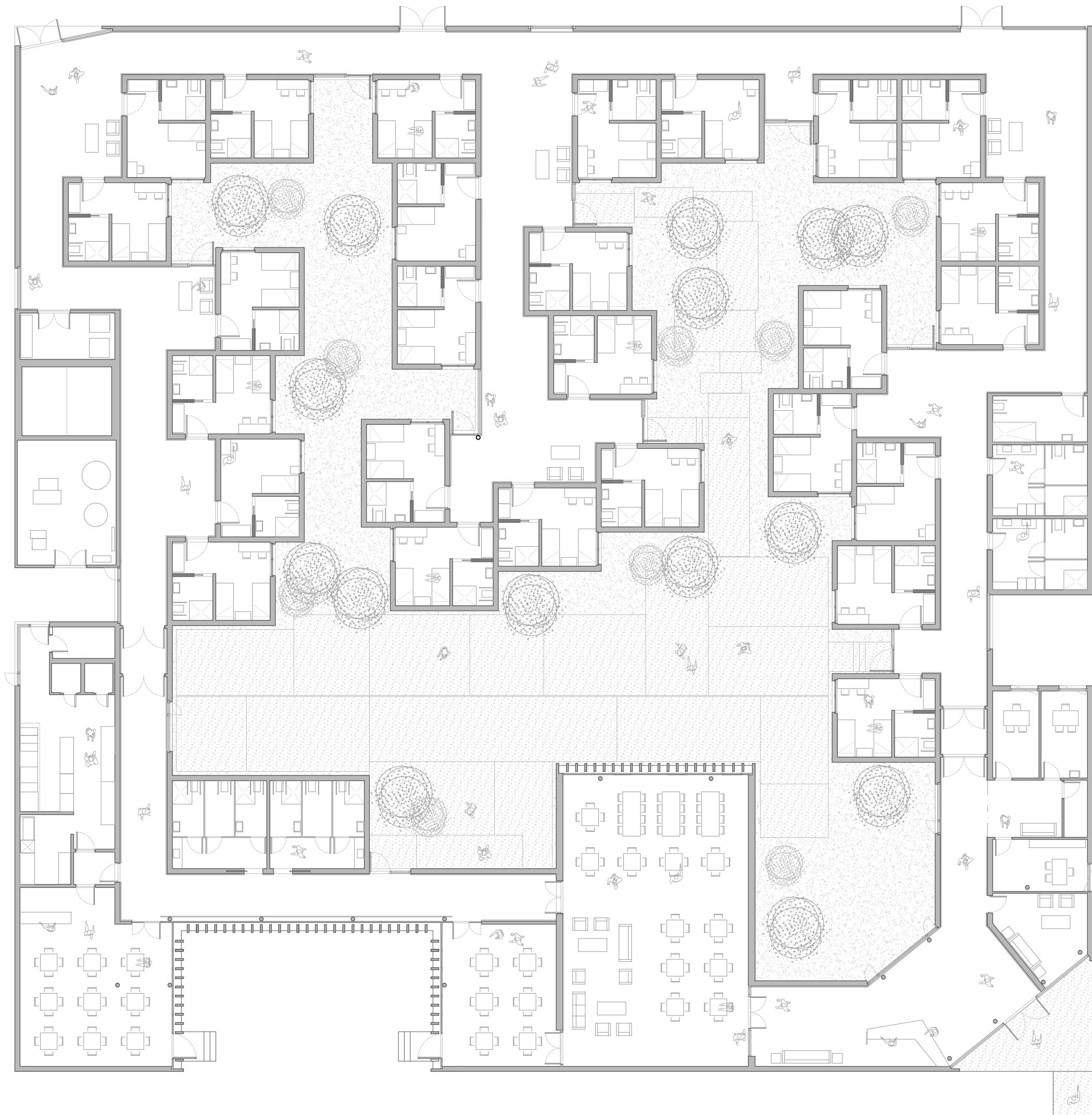
Residencia de mayores en Aldeamayor _ Planta baja ±0.00m
