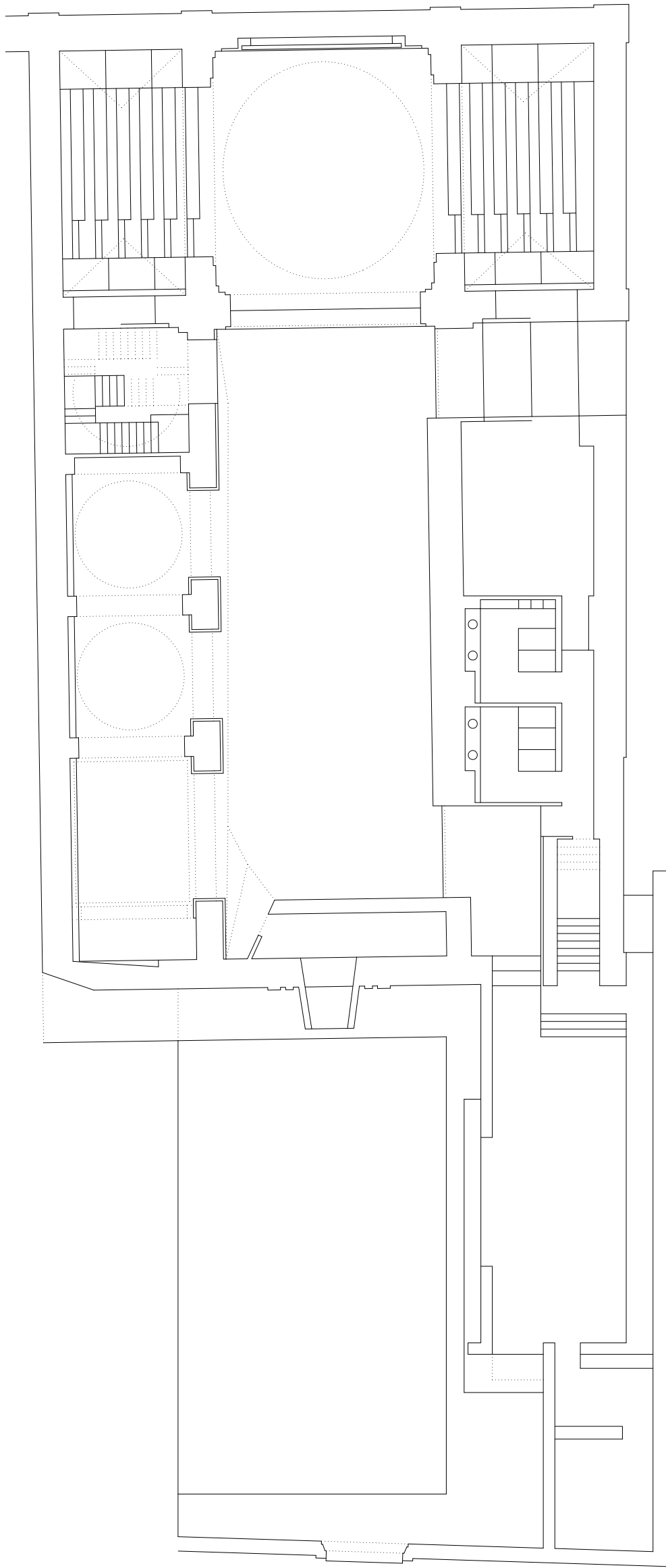
PLANTA BAJA
