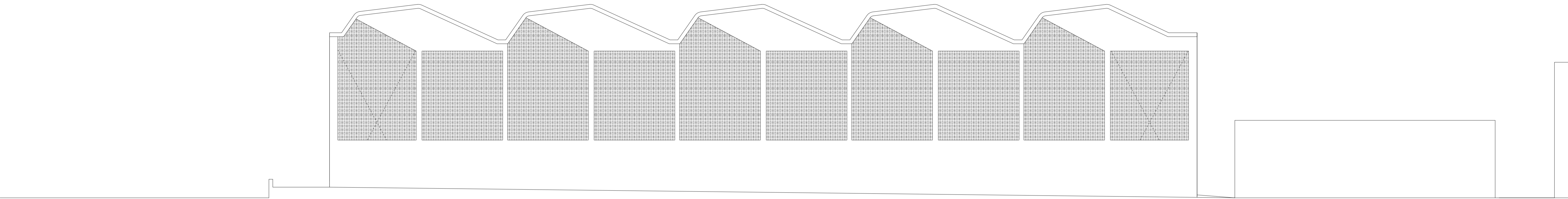
ALZADO OESTE
