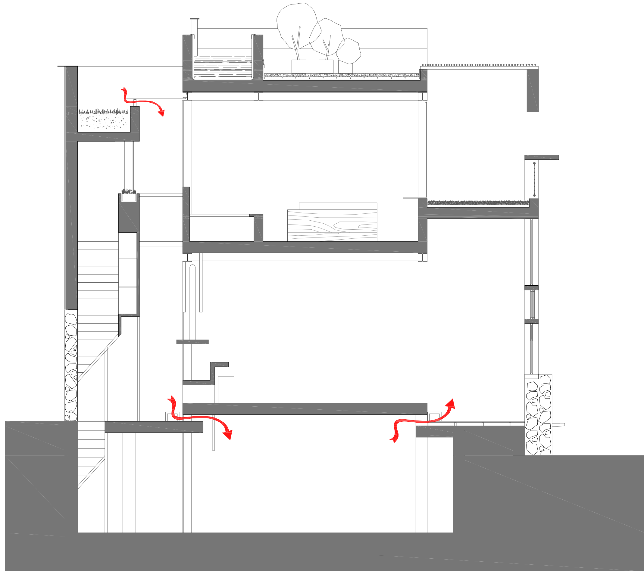
SECCIÓN TRANSVERSAL
