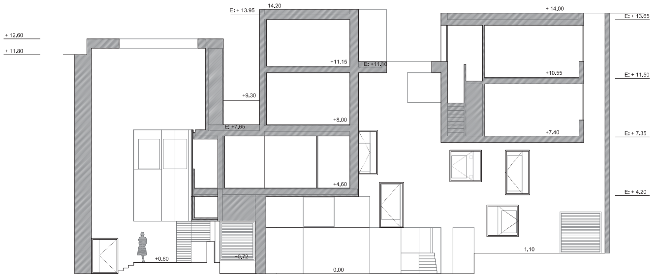
Sección 1-1'
