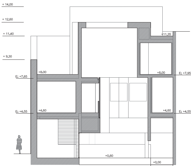
Sección 2-2'
