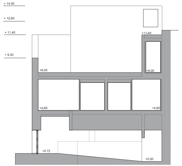
Sección 3-3'
