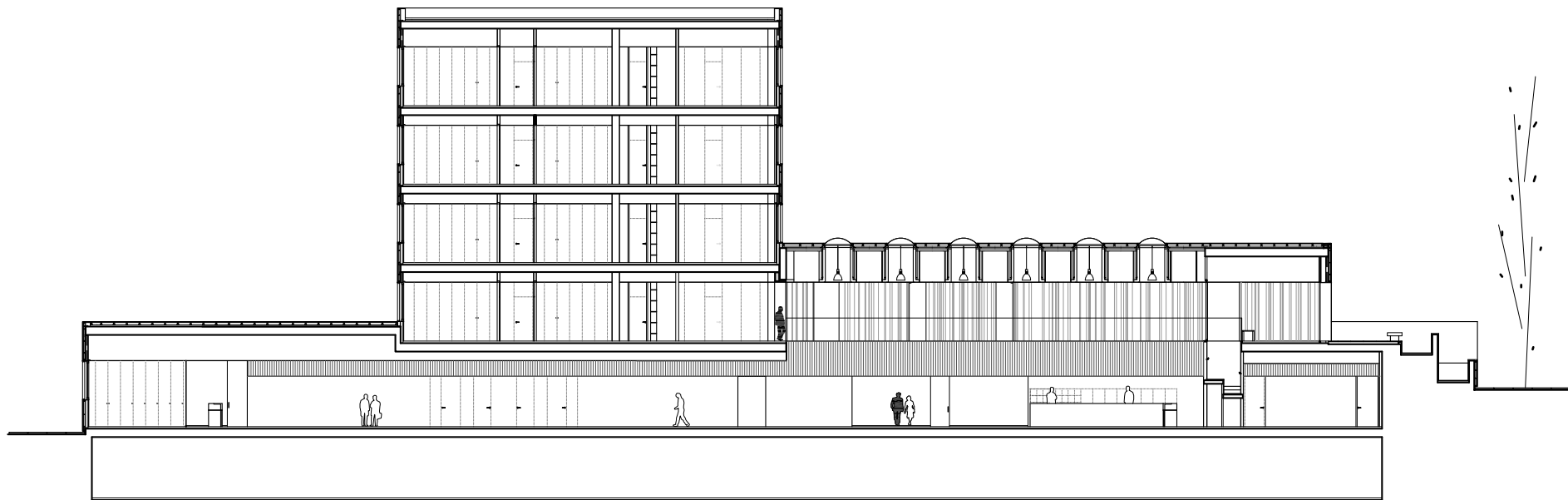
SECCION LONGITUDINAL
