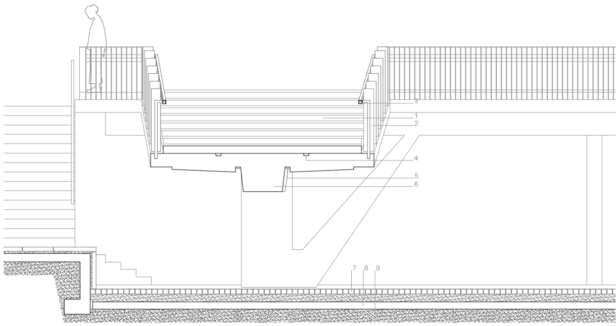
SECCIÓN TRANSVERSAL
