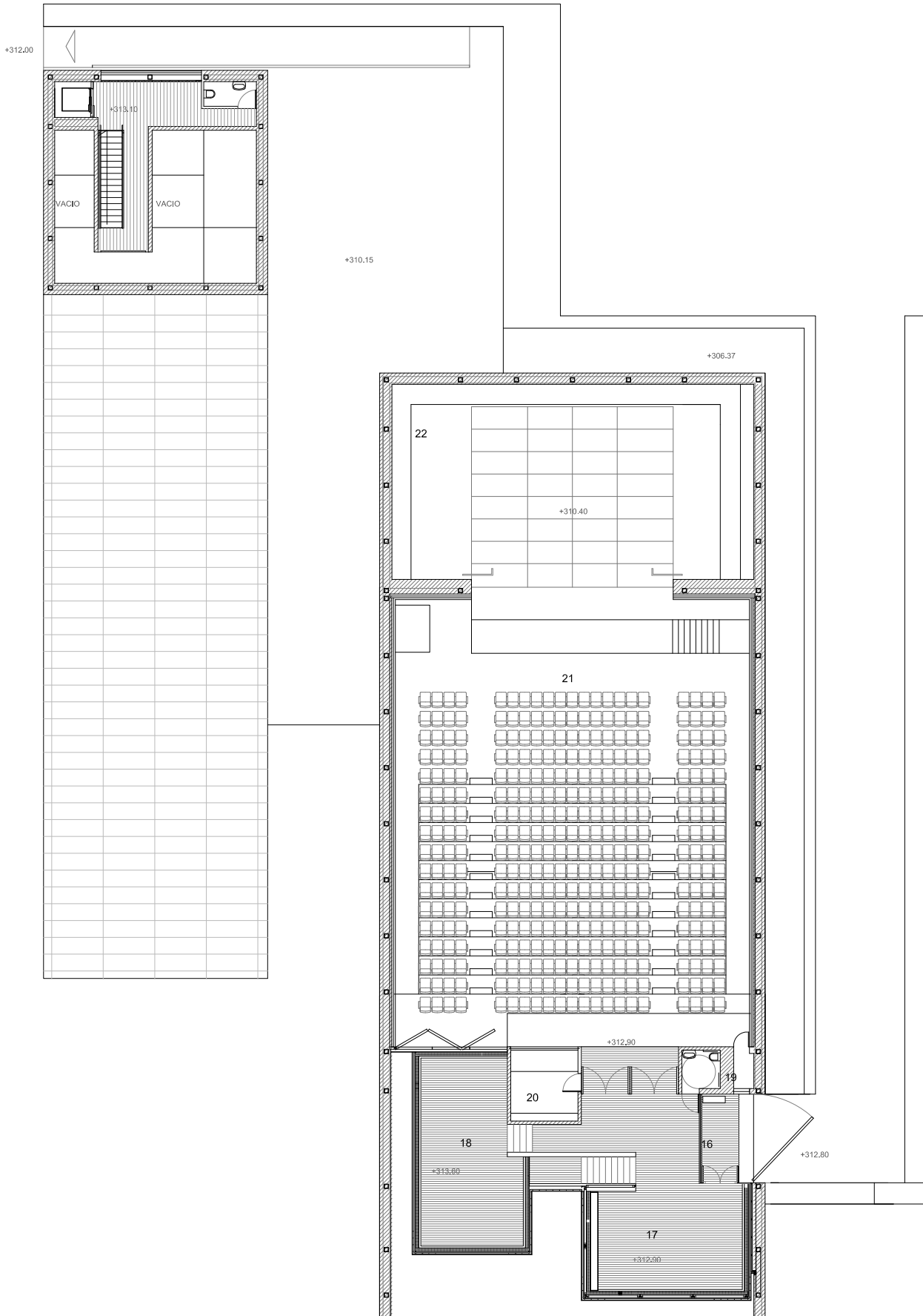
PLANTA COTA +315.60
