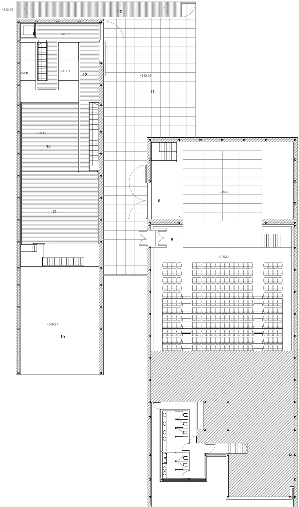
PLANTA COTA +310.85
