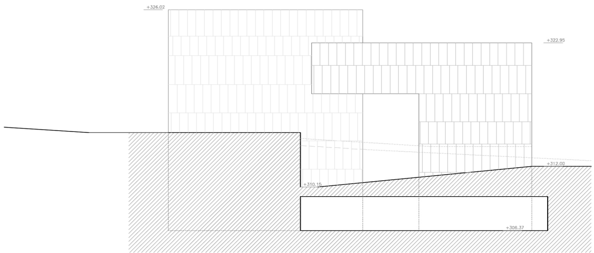
ALZADO TRANSVERSAL DD' 0 5 10 mts.
