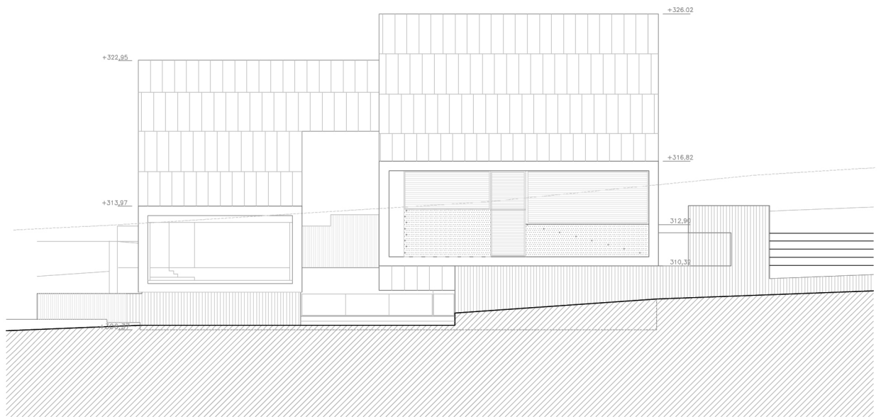
ALZADO TRANSVERSAL AA' 0 5 10 mts.
