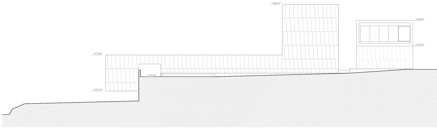
ALZADO LONGITUDINAL AA' 0 5 10 mts.
