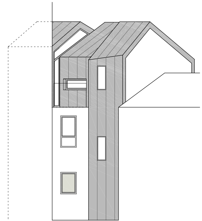
ALZADO PATIO TRASERO (SUR)
