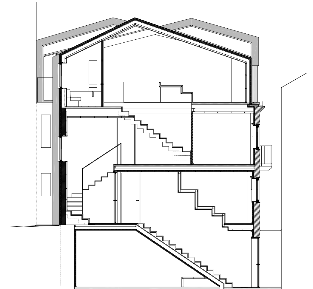
SECCION LONGITUDINAL
