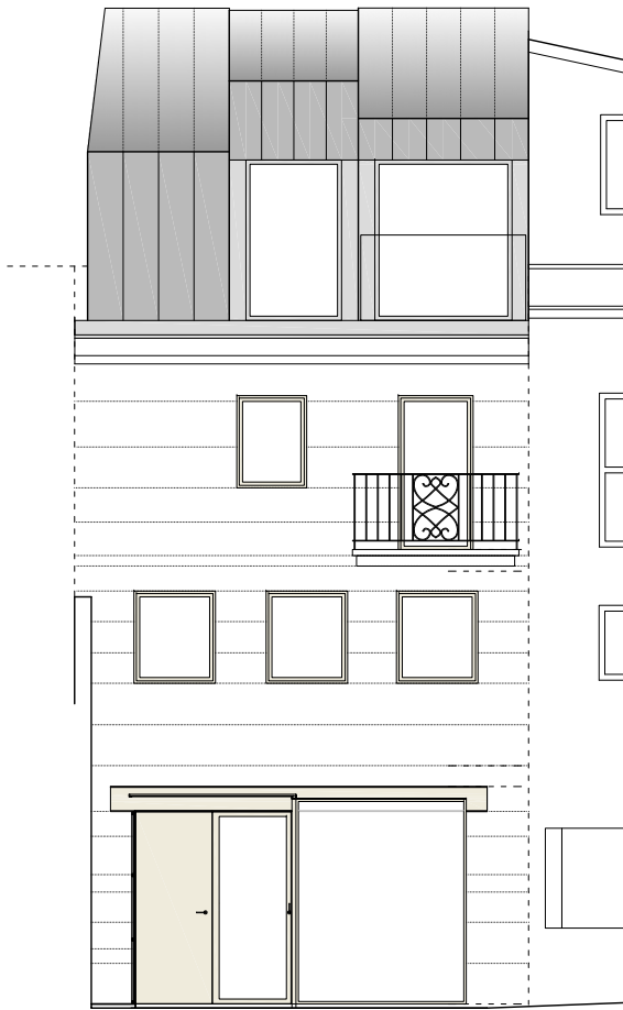
ALZADO CALLE MENDEZ NUÑEZ (NORTE)
