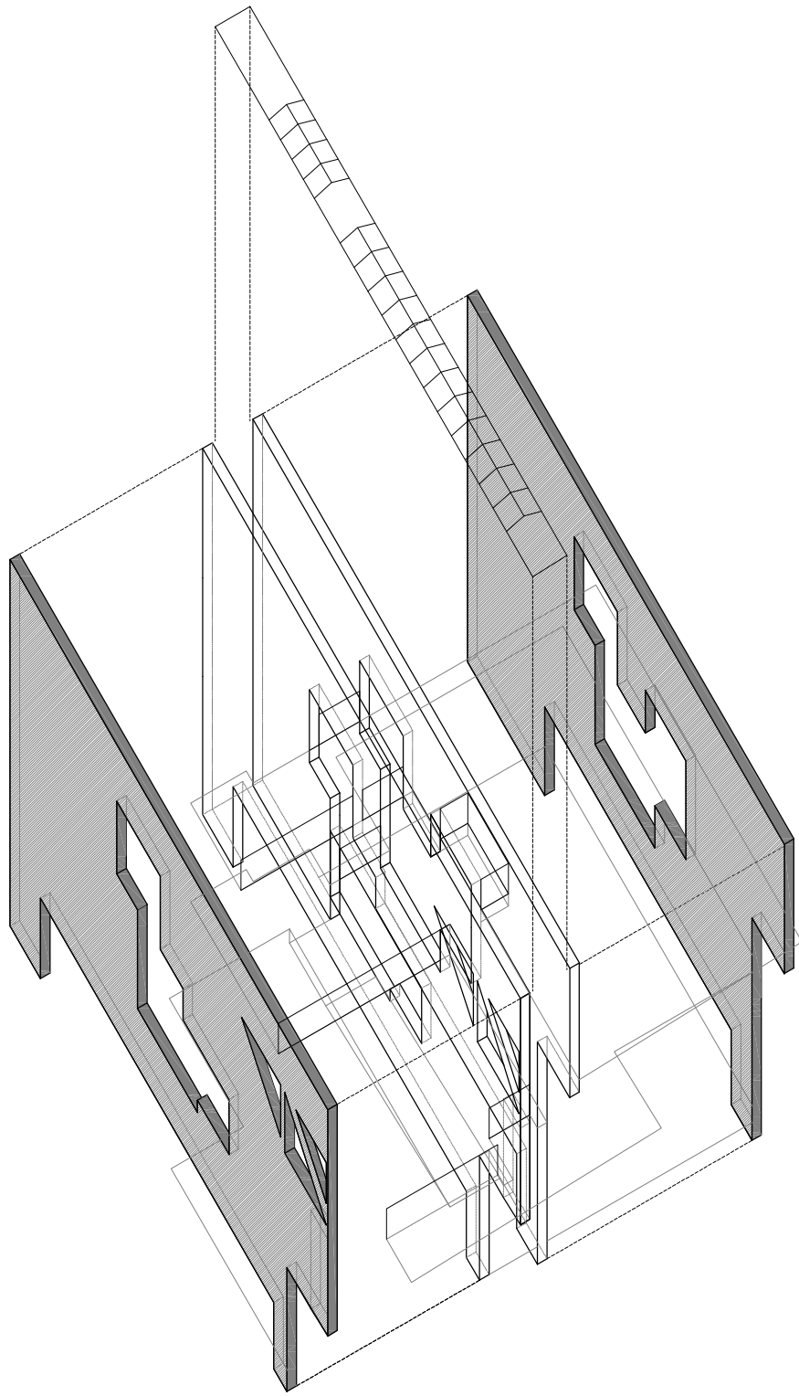
HUECO CENTRAL AXONOMETRÍA
