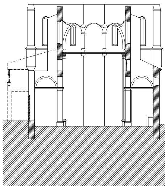
SECCION ESTADO INICIAL
