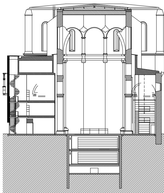
SECCION ESTADO REFORMADO
