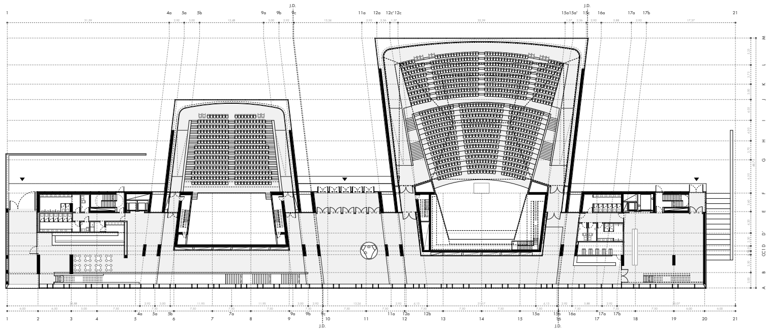
ACCESO PRINCIPAL PLANTA NIVEL 2 cota +9,18 m
