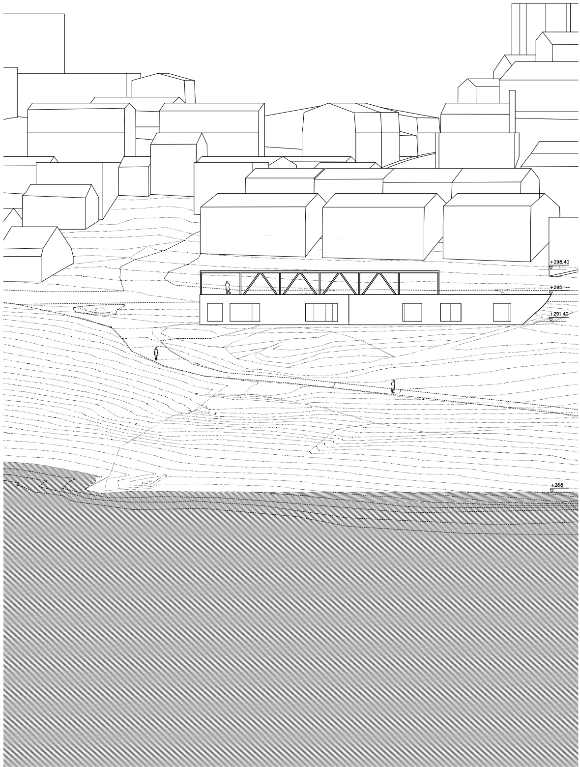
ALZADO GENERAL 0 5 10 25 m
