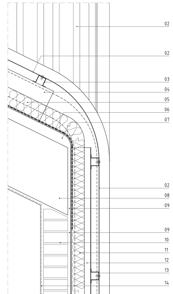
DETALLE ALZADO-SECCION FACHADA EXTERIOR
