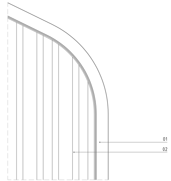
DETALLE ALZADO REMATE SUPERIOR DE FACHADA MEDIANERA CON CUBIERTA. ENCUESTRO EN FACHADA EXTERIOR
