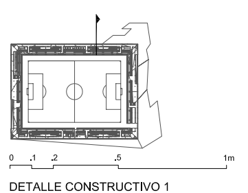
DETALLE CONSTRUCTIVO 1
