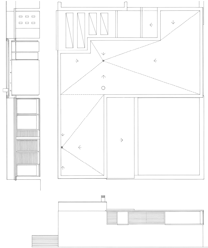
Planta y alzados tipo 3B Urbanización en el Novo Sancti Petri. Chiclana, Cádiz Cruz y Ortiz arquitectos
