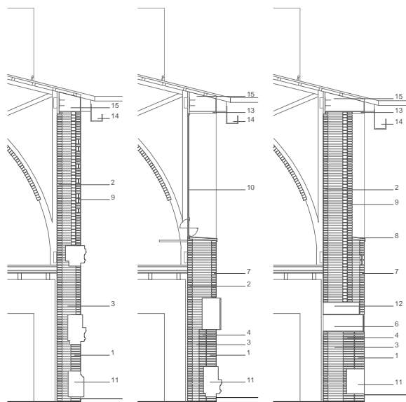
sección vertical E
