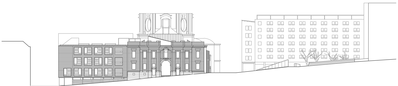
ALZADO A C/ MESÓN DE PAREDES
