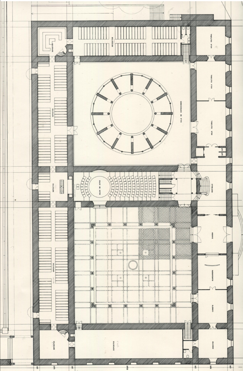
SECCIÓN TRANSVERSAL Y PLANTAS DE ACCESO Y SUPERIOR E1:500
