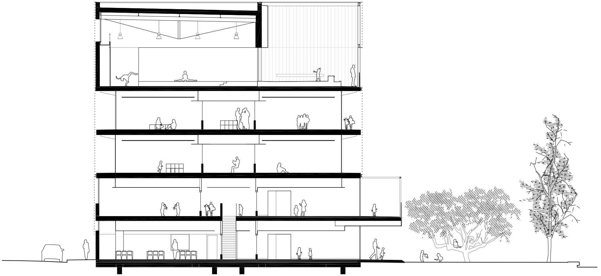
Sección
