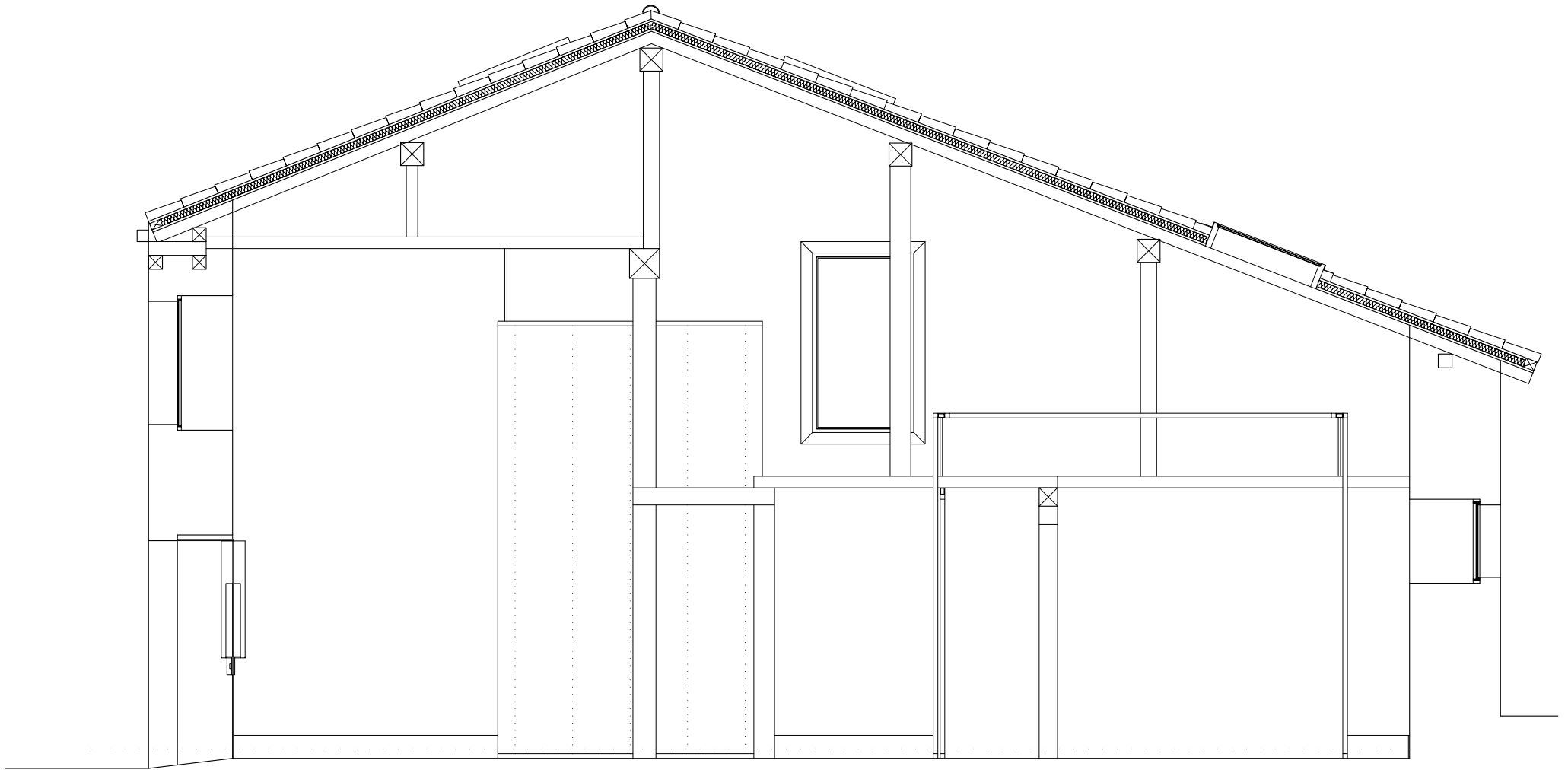
SECCIÓN A-A'
