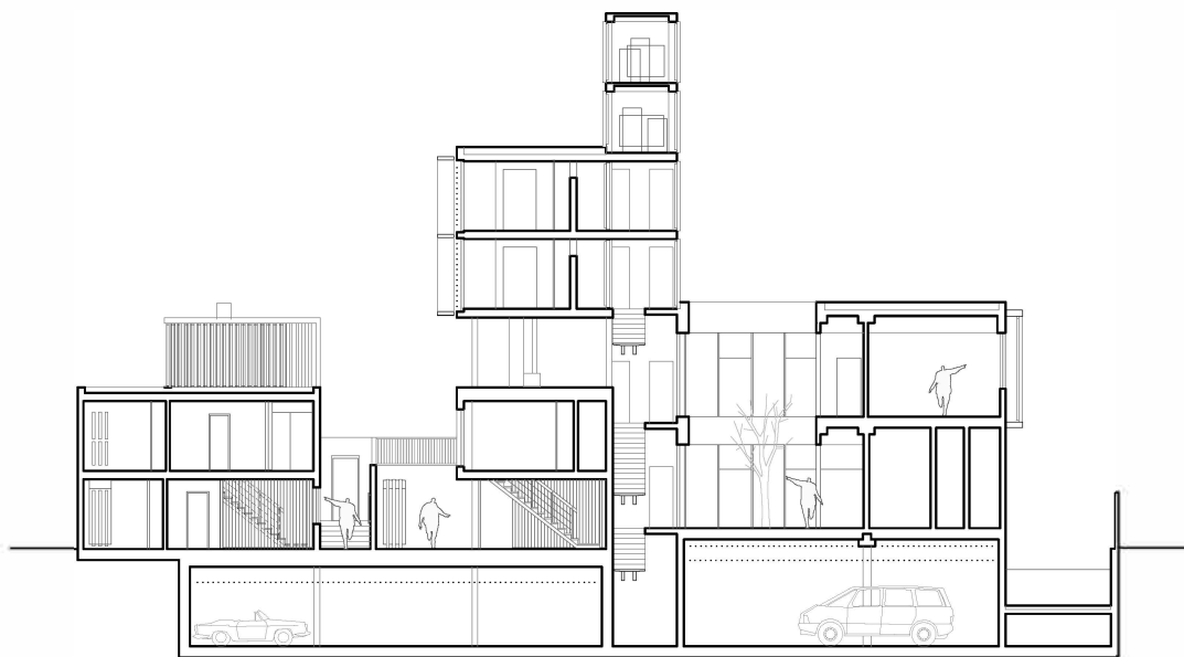
sección b-b'
