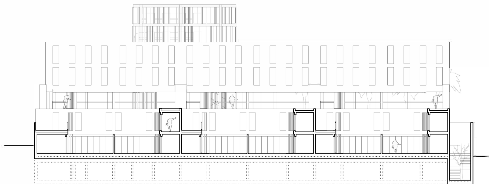
sección c-c'
