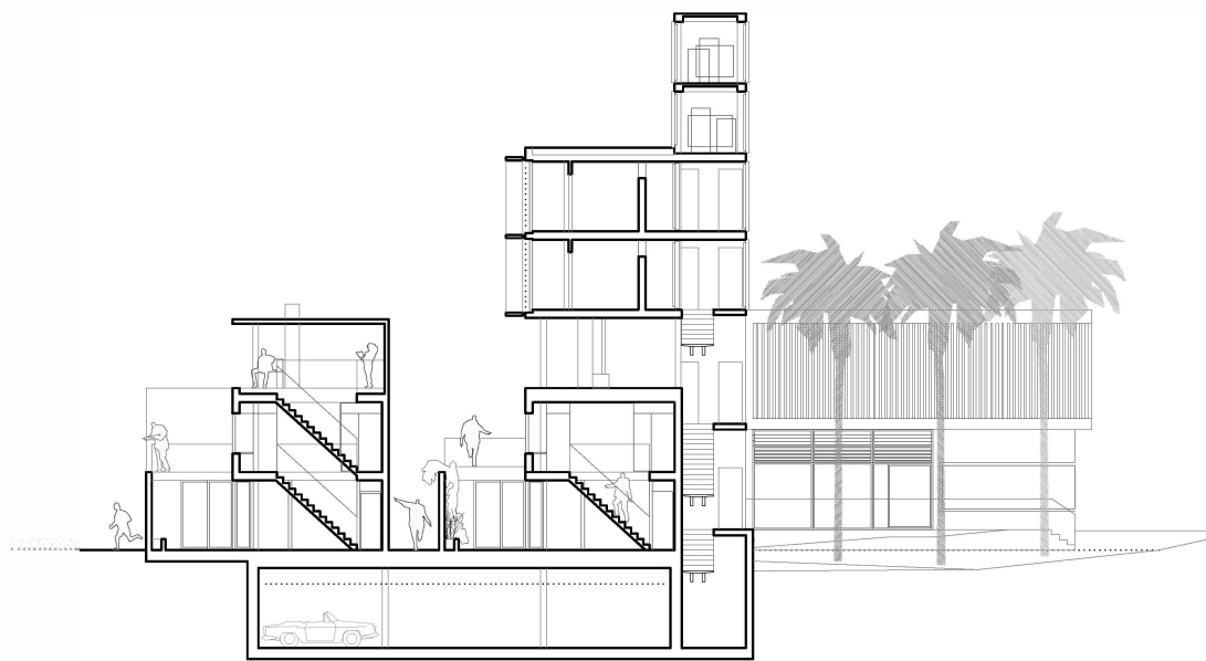
sección a-a'
