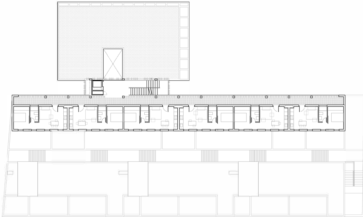
planta 3 a y 4 a apartamentos
