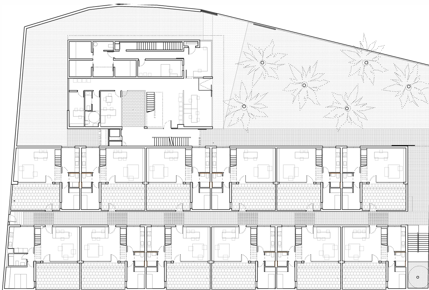
planta baja viviendas y oficinas
