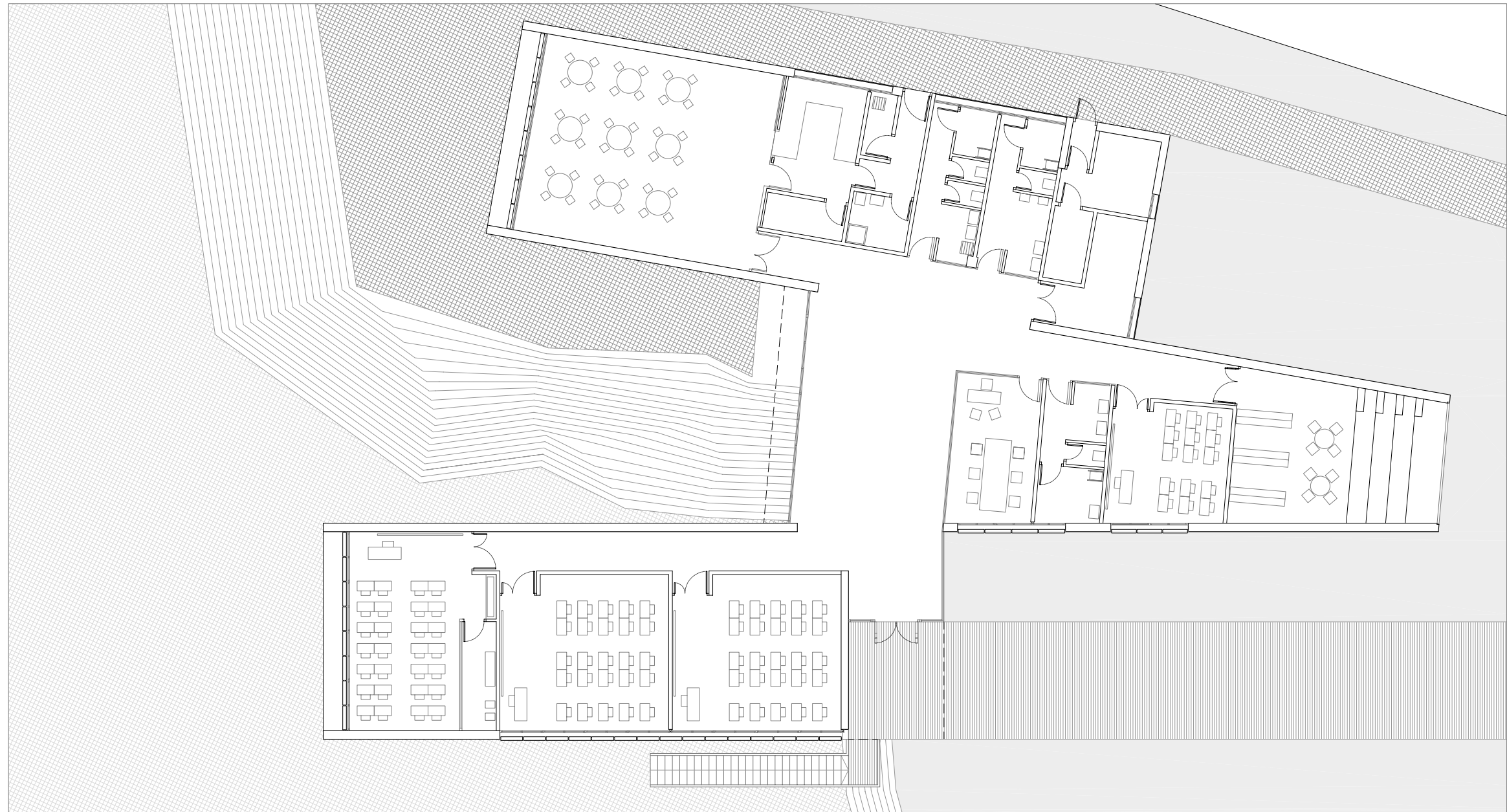
Planta cota +0,15m
