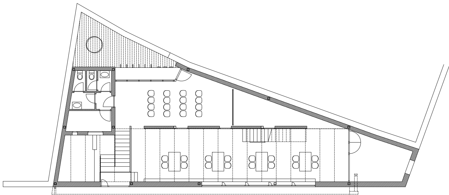
planta primera
