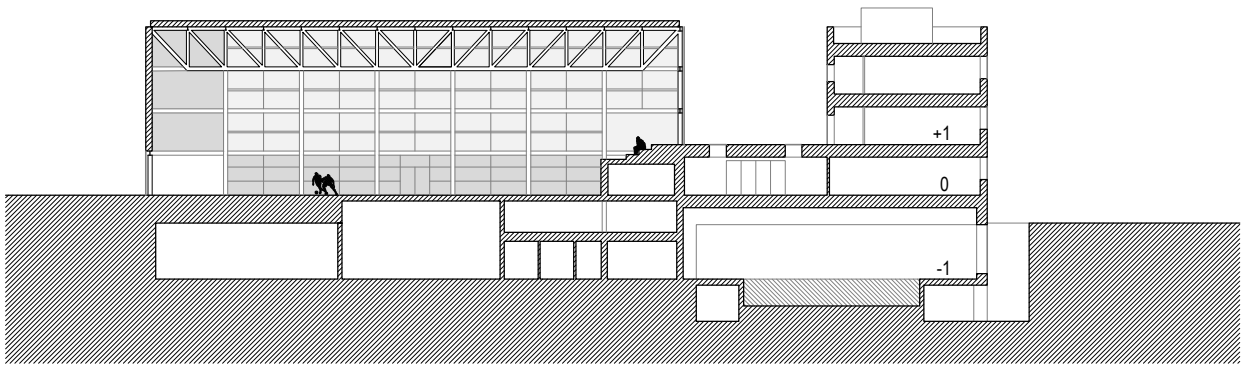
LONGITUDINAL SECTION
