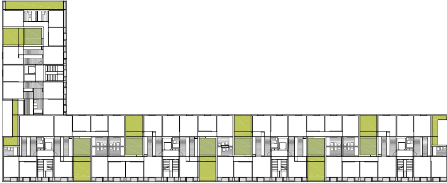
EDIFICIO 01. P. SEGUNDA (+75.05) / P. CUARTA (+81.60). E:1/300
