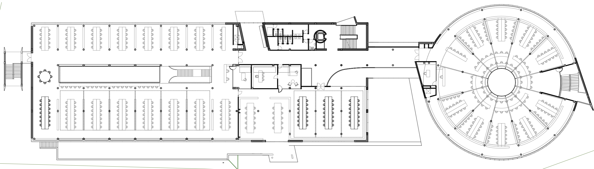
PLANTA SEGUNDA
