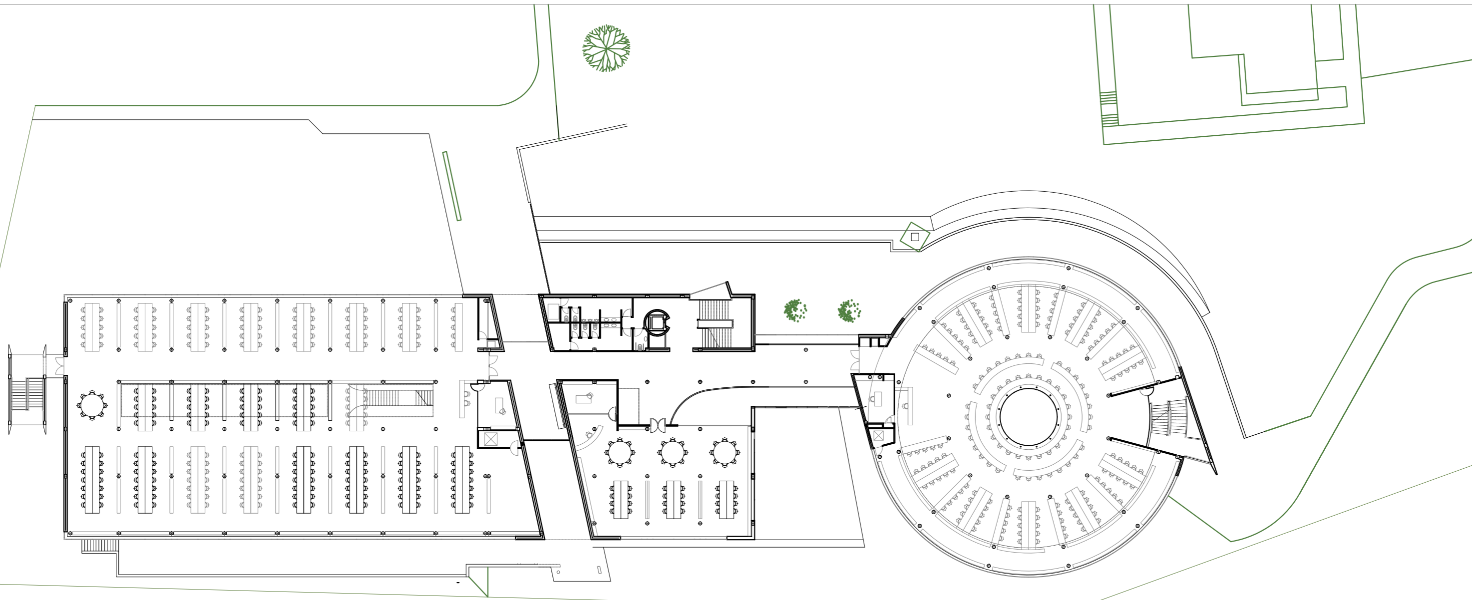
PLANTA PRIMERA
