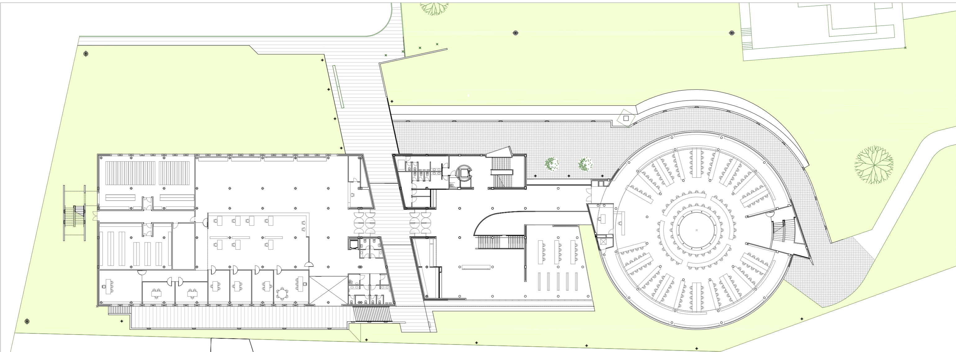
PLANTA BAJA. ACCESO
