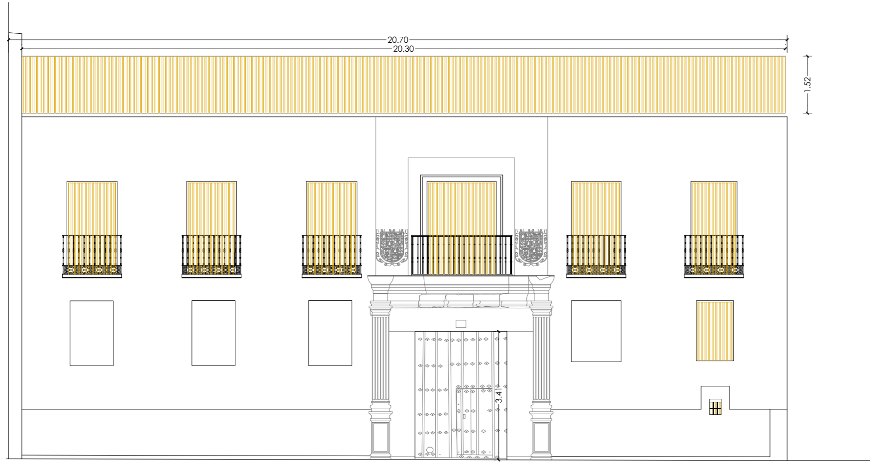
ALZADO ESTE
