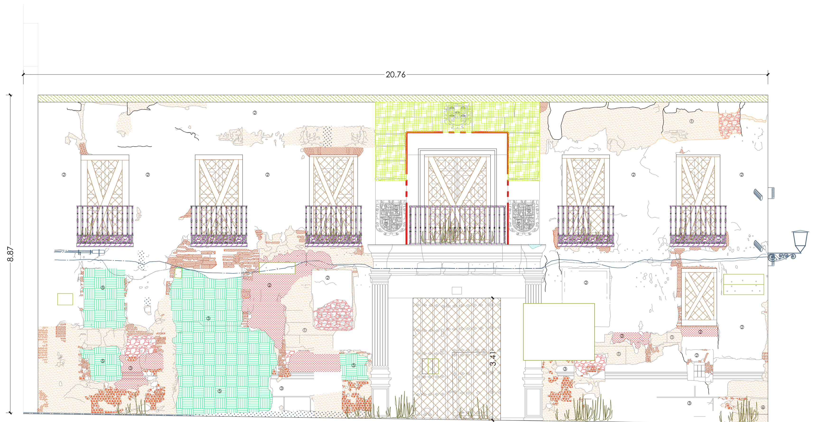
ALZADO ESTE
