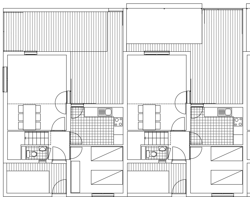
planta baja
