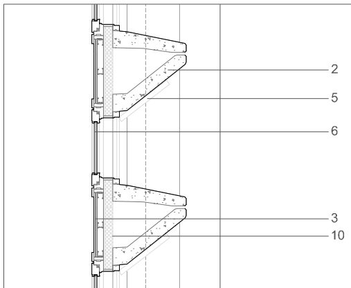
DETALLE DE PREFABRICADO DE HORMIGÓN ARMADO
